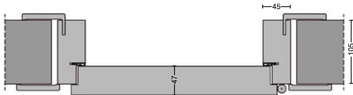
Porta EI 45 Fonoisolante 32 dB - 35,5 dB
