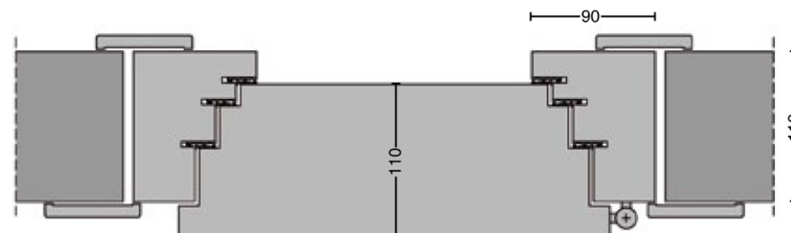
Porta EI 120 Fonoisolante 46 dB
