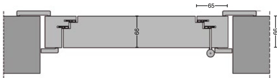
Porta EI 30/60 Complanare - Fonoisolante 40 dB
