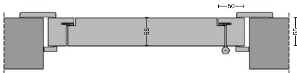
Porta EI 30/60 Complanare - Fonoisolante 32 dB - 36 dB
