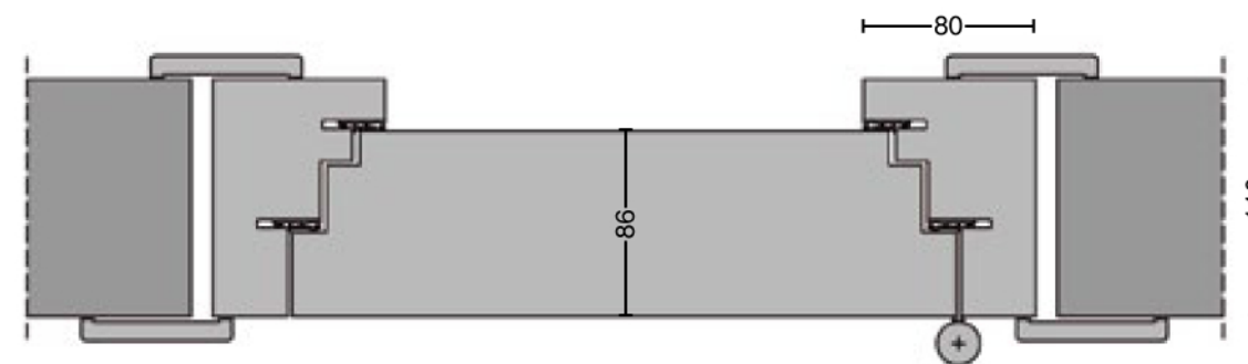
Porta EI 120 Fonoisolante 43 dB
