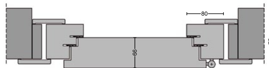
Porta REI 60 Fonoisolante 40 dB
